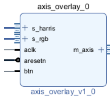
FIGURE 8 : BLOC IP DE L'OVERLAY
